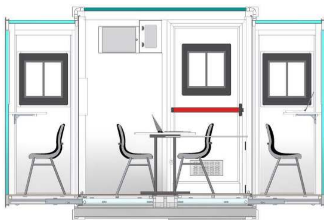
Vertikalschnitt des „erweiterten“ Moduls
