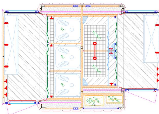
Disegno Pianta del modulo "espanso" in posizione operativa
