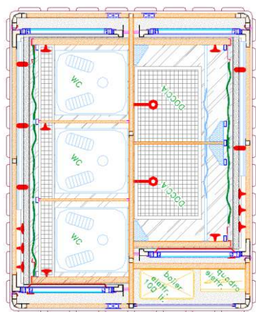
Disegno Pianta del modulo "chiuso"
